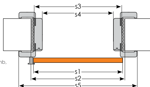
AZ AJTÓLAP ÉS A TOK MÉRETE A FAL ELŐTT TOLÓ
