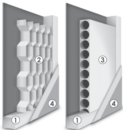
KERESZTMETSZETI RAJZ FÓLIÁS AJTÓK
