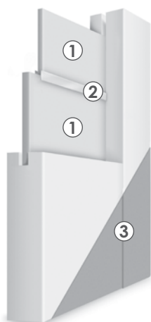
KERESZTMETSZETI RAJZ MODUL AJTÓK SALENTO
